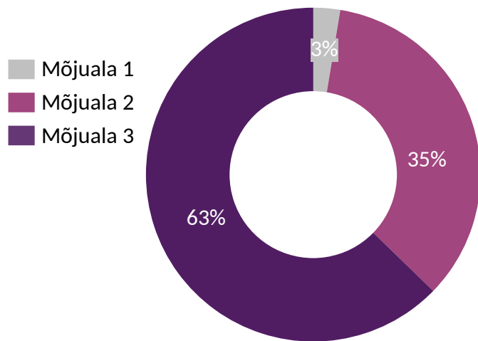
JOONIS 2. PÕLVA HAIGLA KHG JALAJÄLJE JAGUNEMINE MÕJUALADE LÕIKES (%)
