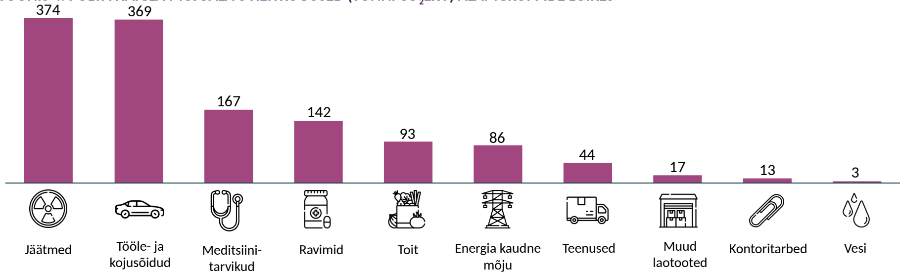
JOONIS 4. PÕLVA HAIGLA MÕJUALA 3 HEITKOGUSED (TONNI CO 2 EKV) ALAMGRUPPIDE LÕIKES
