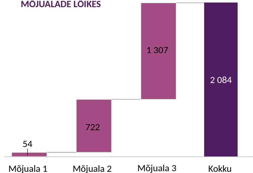
JOONIS 3. PÕLVA HAIGLA KHG JALAJÄLG (TONNI CO 2 EKV) MÕJUALADE LÕIKES
