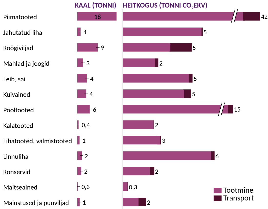
JOONIS 6. TOIDUKAUPADE KOGUS JA TOOTMISE JA TRANSPORDI HEITKOGUSED
