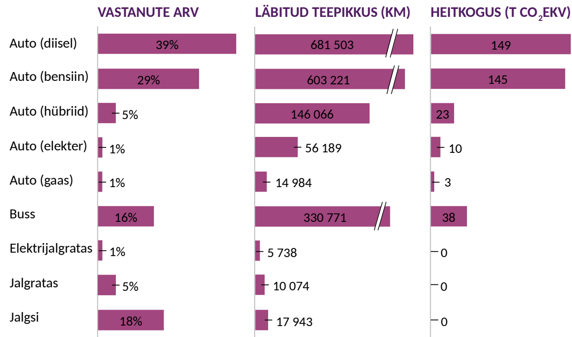
JOONIS 5. TÖÖLE- JA KOJUSÕITUDE KÜSITLUSE TULEMUSED JA KHG JALAJÄLG
